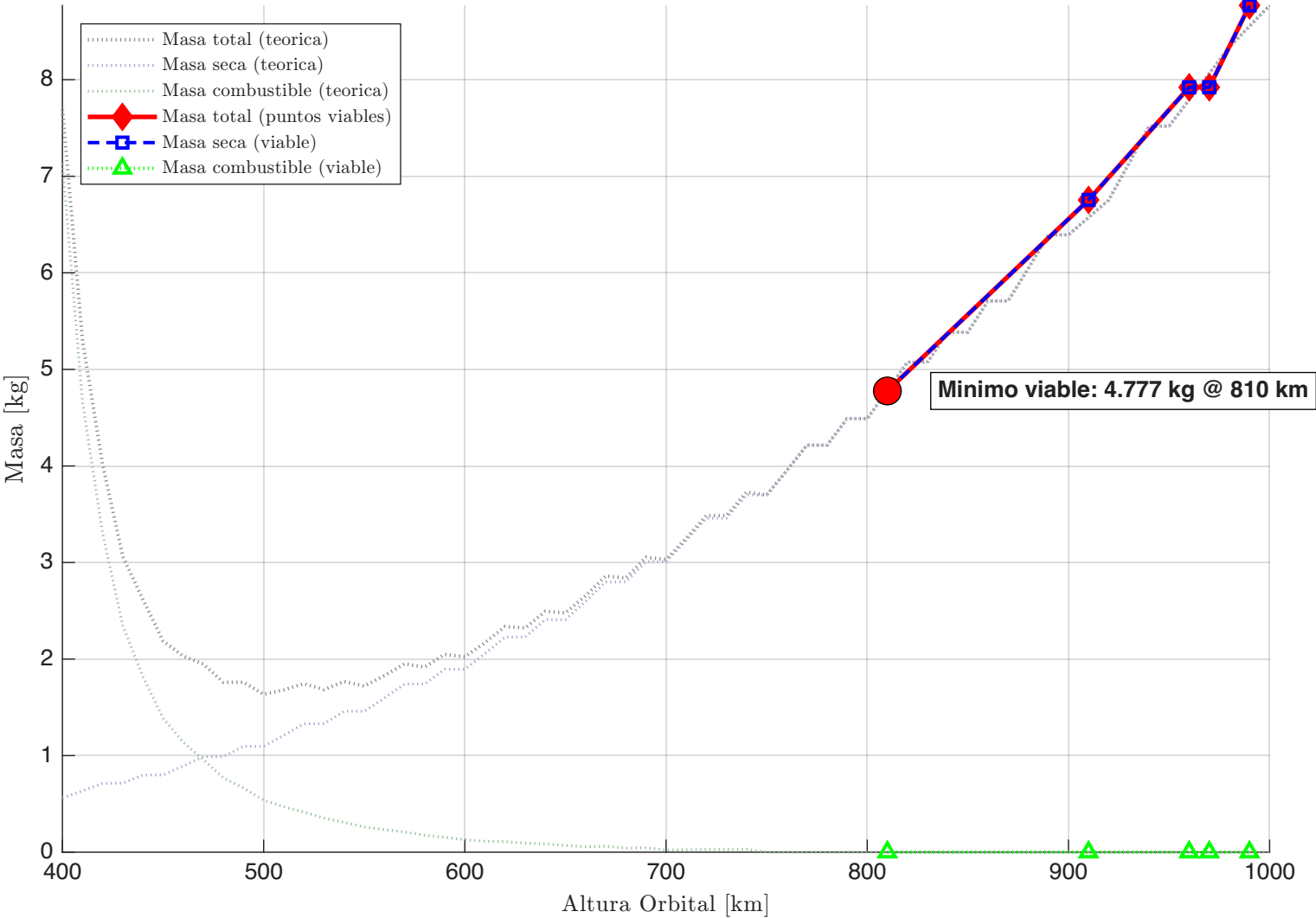
Desglose de Masas vs. Altura Config: 3 Sat, 1 Tel, Det 3, Refractivo
